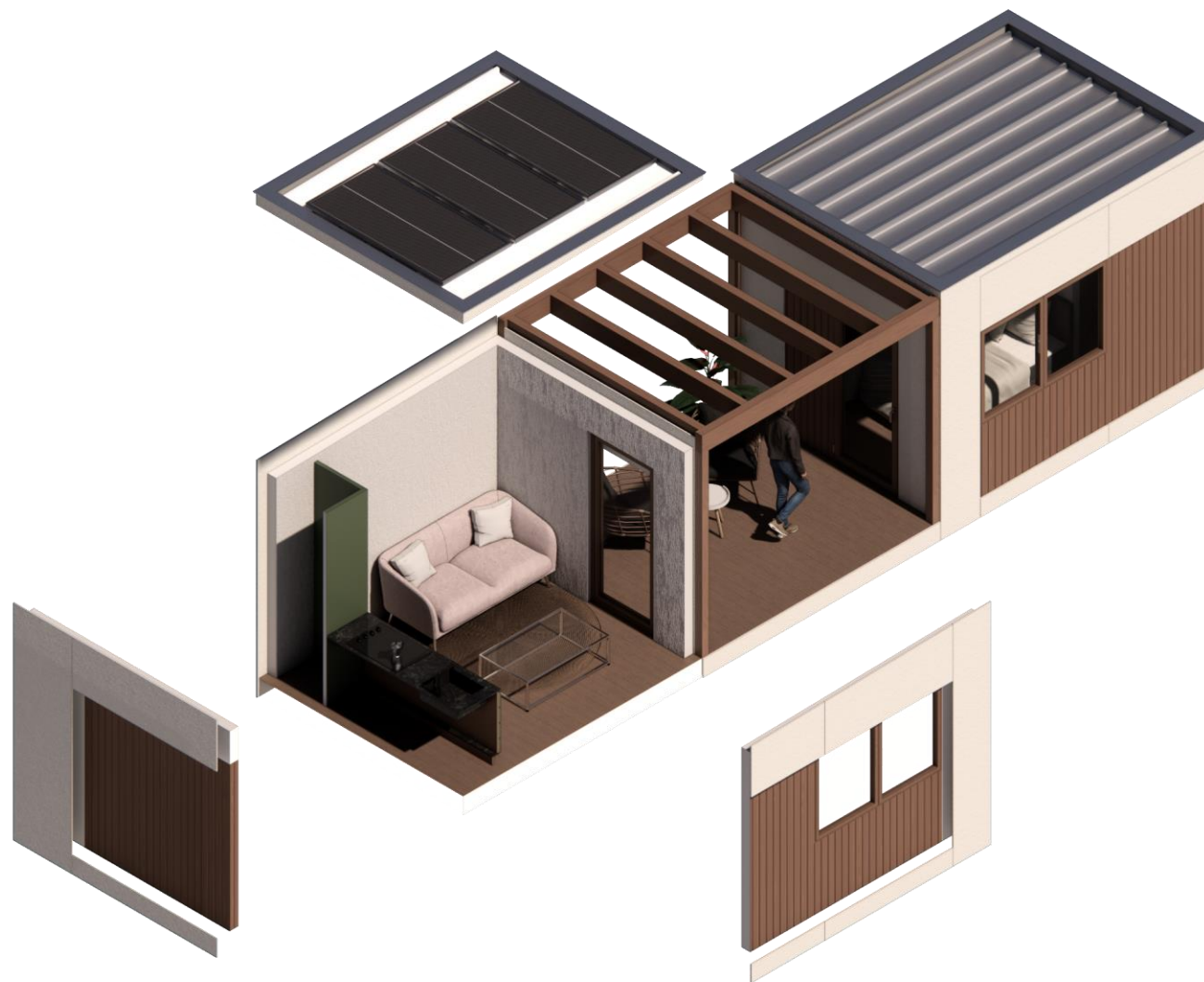
AXONOMETRÍA EXPLOTADA SIN ESTRUCTURA MÓDULO 3x3'5 m
