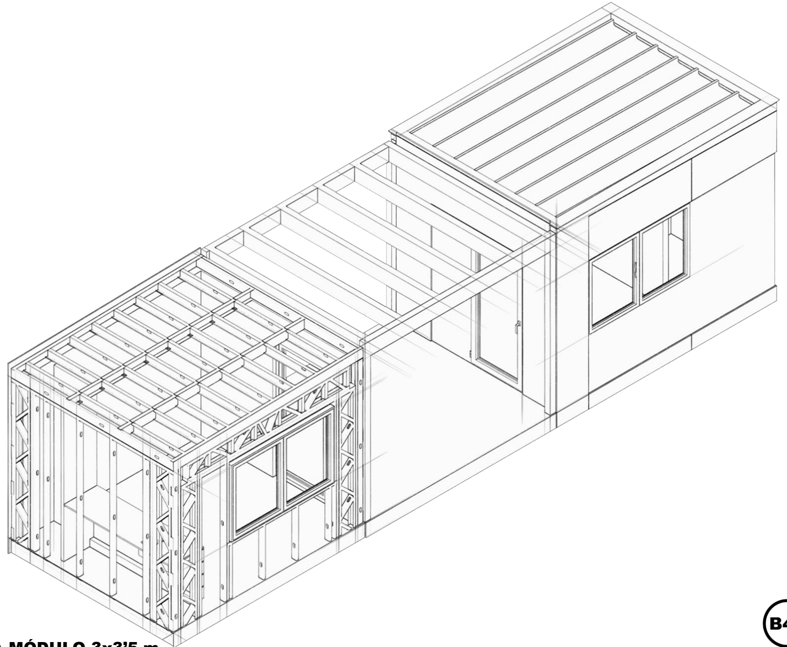
AXONOMETRÍA MÓDULO 3x3'5 m
