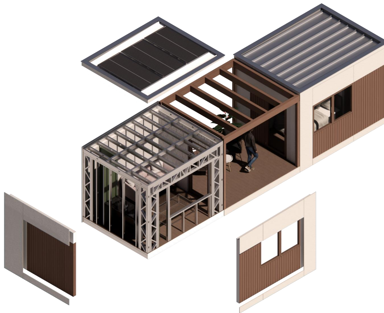
AXONOMETRÍA EXPLOTADA MÓDULO 3x3'5 m
