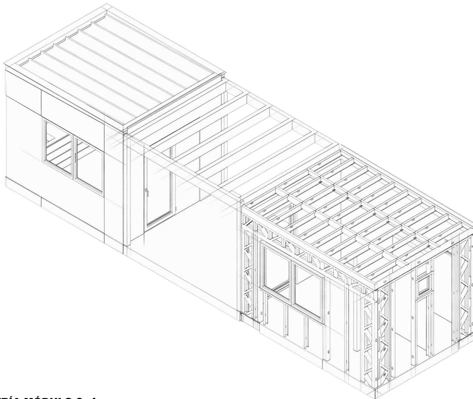
AXONOMETRÍA MÓDULO 3x4 m
