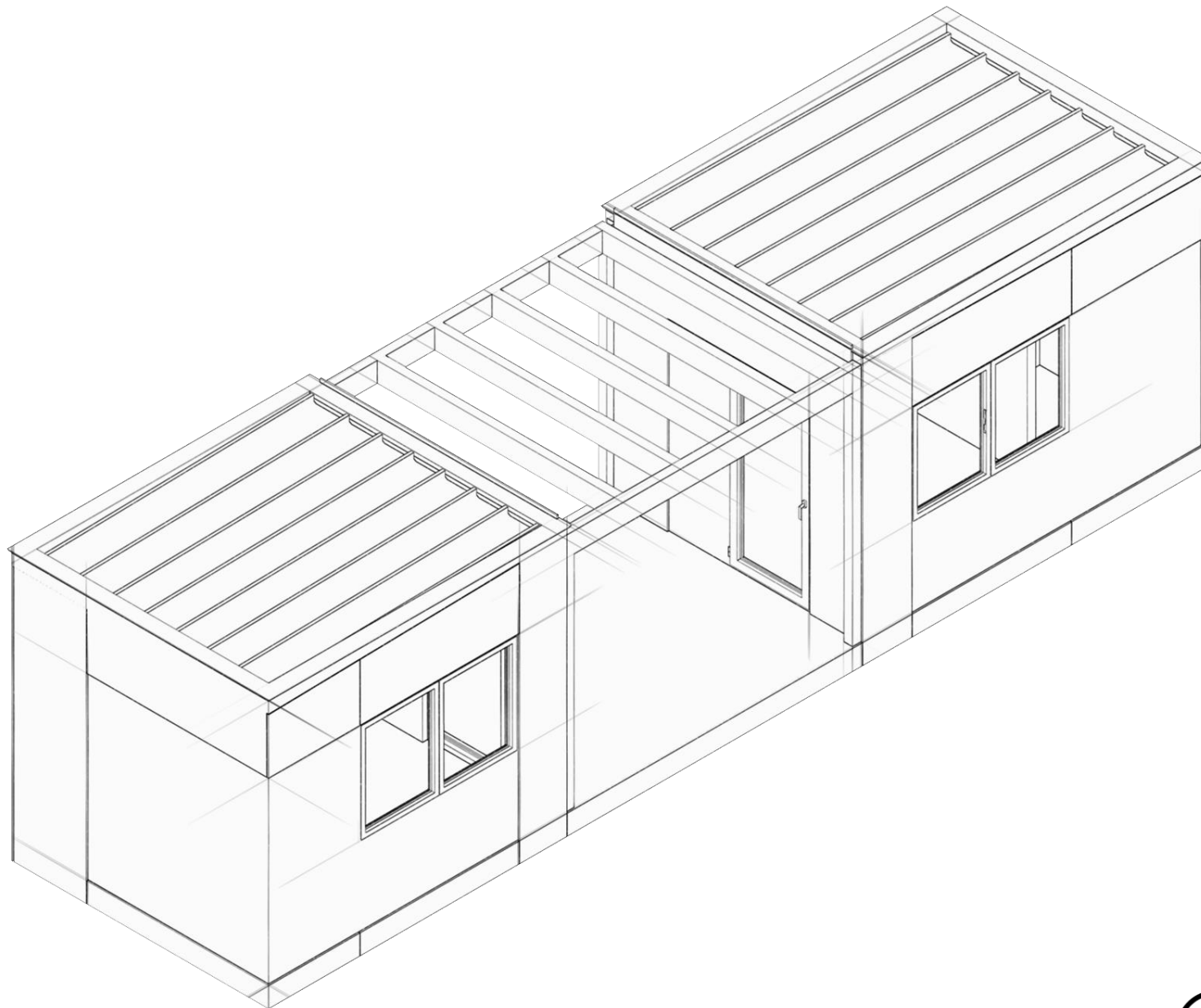
AXONOMETRÍA COMPLETA DELANTERA
